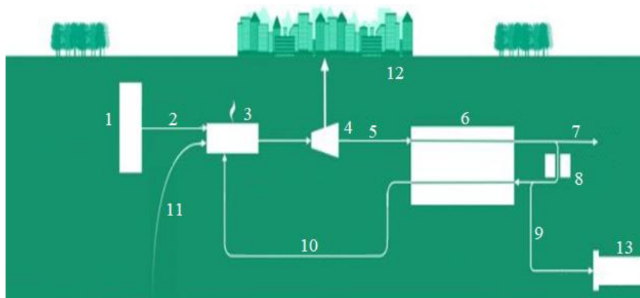
Рис. 2. Схема, поясняющая технологический процесс ТЭС: 1 – блок разделения воздуха и выделения из него чистого кислорода; 2 – чистый кислород; 3 – камера сгорания; 4 – газовая турбина; 5 – смесь «вода–диоксид углерода»; 6 – теплообменник; 7 – сточные воды; 8 – насосы; 9 – диоксид углерода, поступающий под землю; 10 – диоксид углерода, поступающий в камеру сгорания как вторичное топливо; 11 – топливо; 12 – здание ТЭС
